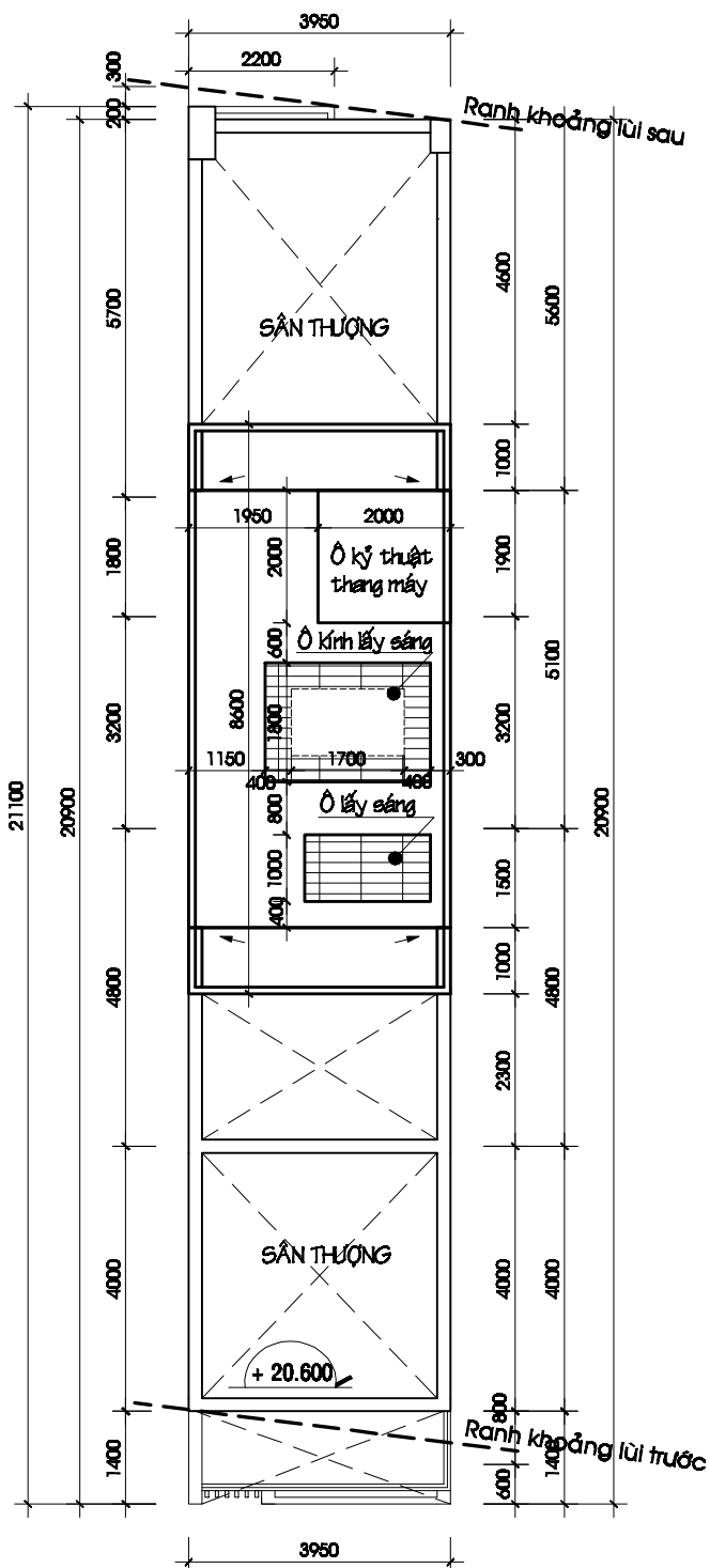
● MẶT BẰNG MÁI TL : 1/ 100
