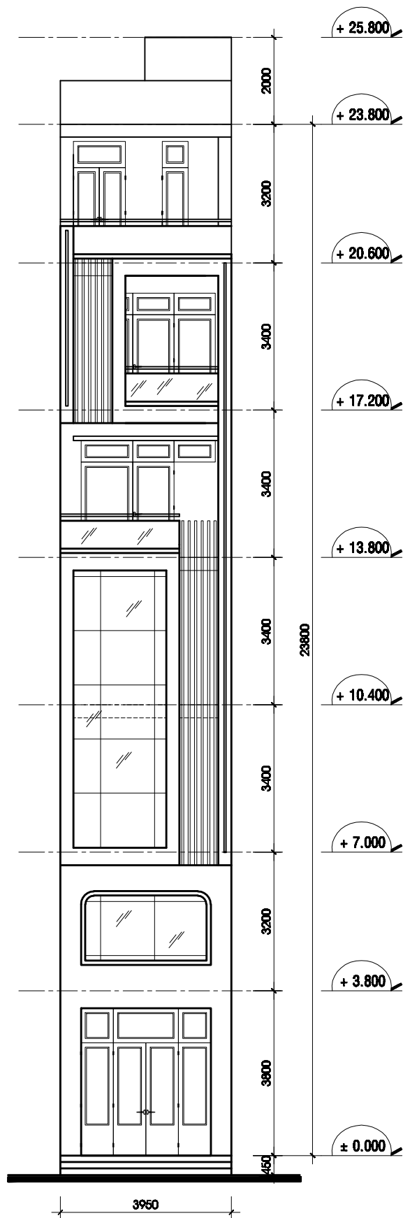
● MẶT ĐŨNG CHÍNH TL : 1/ 100
